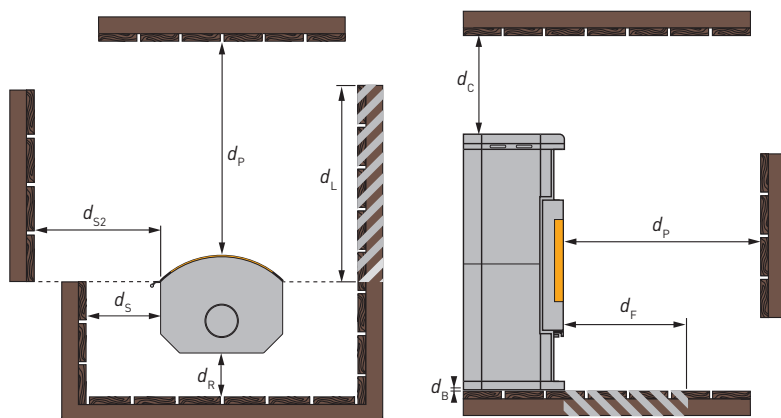
Draufsicht Brennkammer
